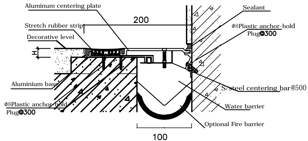
MSD-QSJ 100mm
